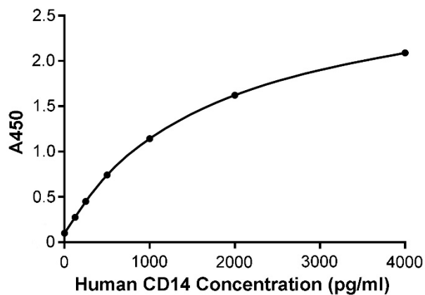
图3. Human CD14 ELISA Kit的标准曲线。实测数据会因实验条件、检测仪器等的不同而存在差异，图中数据仅供参考。
